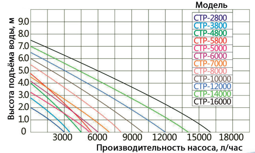
Диаграммы производительности насосов серии СТР-1000
